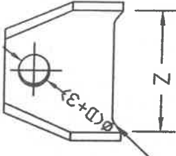
מצמד 2-2
