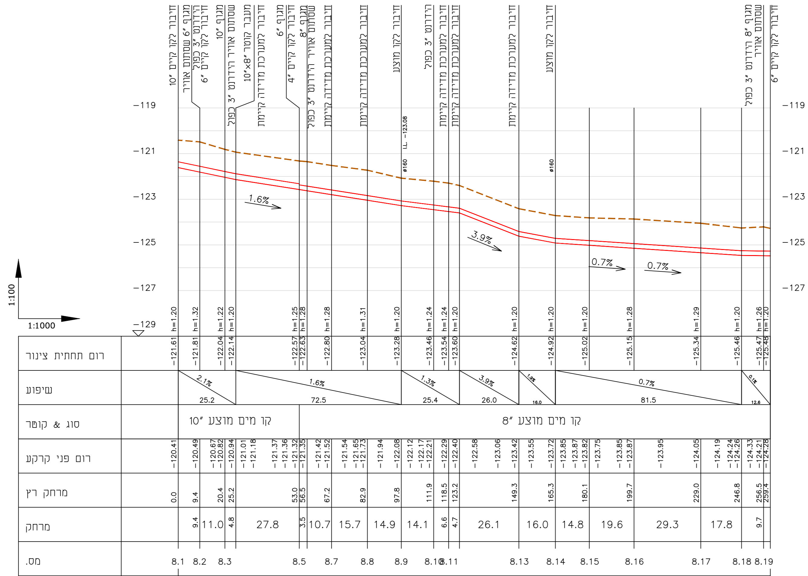
8 קו מים מוצע - קו צינור: 8
